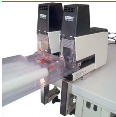
Doppelheftung mit Tischzwingen
